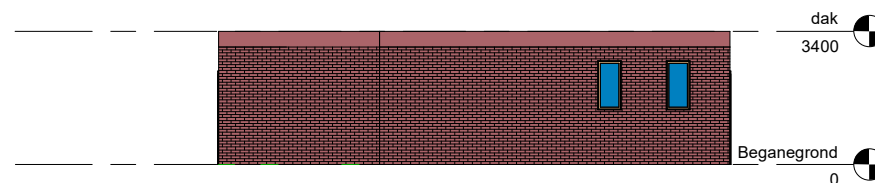
4 Zijkant rechts 1 : 100
